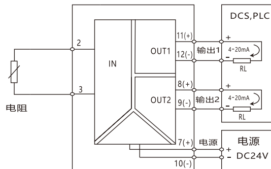
TB-R2XX 一入二出 TB-R1XX 一入一出仅包含通道1部分
