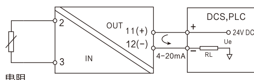
TB-R1X0 一入一出(回路供电)
