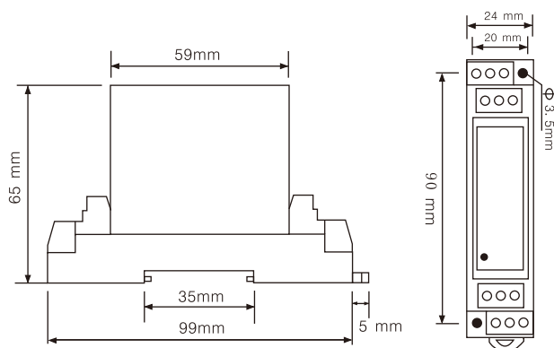
正视图
